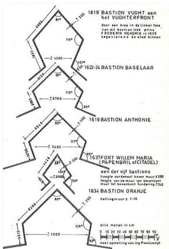
Afbeelding 1.3: De verschillende vormen en afmetingen van de bastions of bolwerken van de vesting 's-Hertogenbosch.
