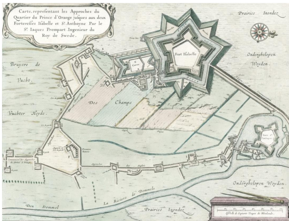
Afbeelding 6.4: De aanvallen op de forten Isabella en Sint Anthonie. De Fransen groeven een weg naar het hoornwerk van het grote fort terwijl de Engelsen de naderingswerkzaamheden richting het kleine fort voor hun rekening namen. Voor de bastions, waar de belegeraars uiteindelijk toesloegen, geldt dat ze voor beide forten nog herkenbaar in het landschap aanwezig zijn.
