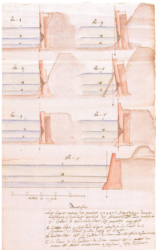
Afbeelding 1.1: Tekeningen uit 1614 van Bollyn en Van Thienen waarop de toestand van de walprofielen is vastgelegd. Naast de uit het lood staande en beschadigde muren, zijn ook de gemiddelde, laagste en hoogst bekende waterstanden getekend.
