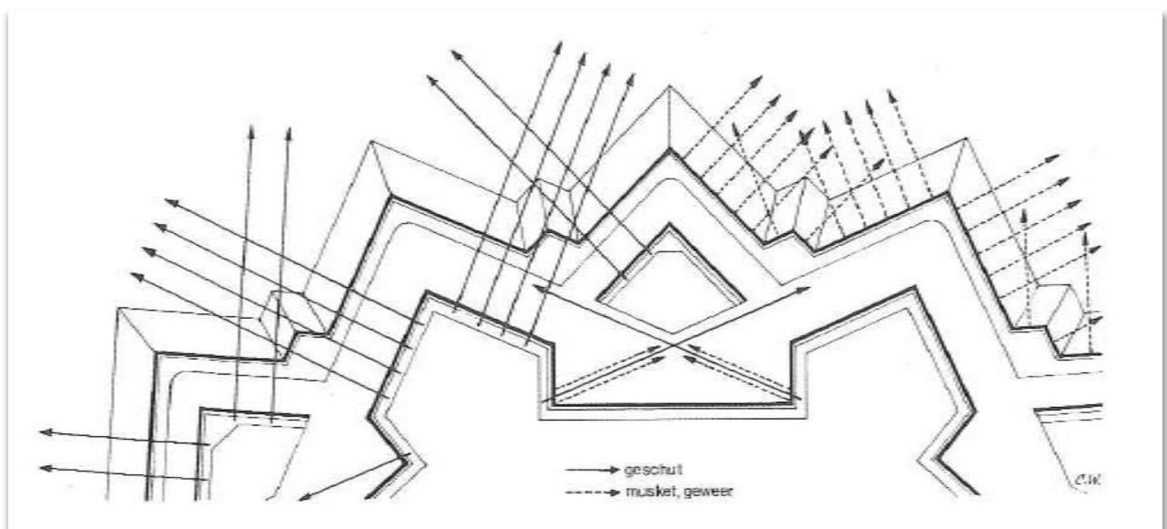
Afbeelding: Hoofdschootsrichtingen vanaf een gebastioneerd vestingwerk.
