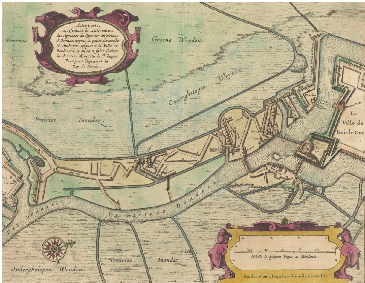
Afbeelding 8.4: De naderingswerkzaamheden voor bastion Vught aan beide zijden van de Dommel. De werken die werden verricht om het halve maanwerk voor de Vughterpoort in handen te krijgen en de galerijen die richting het bastion werden gestuurd, zijn op deze kaart duidelijk zichtbaar.
